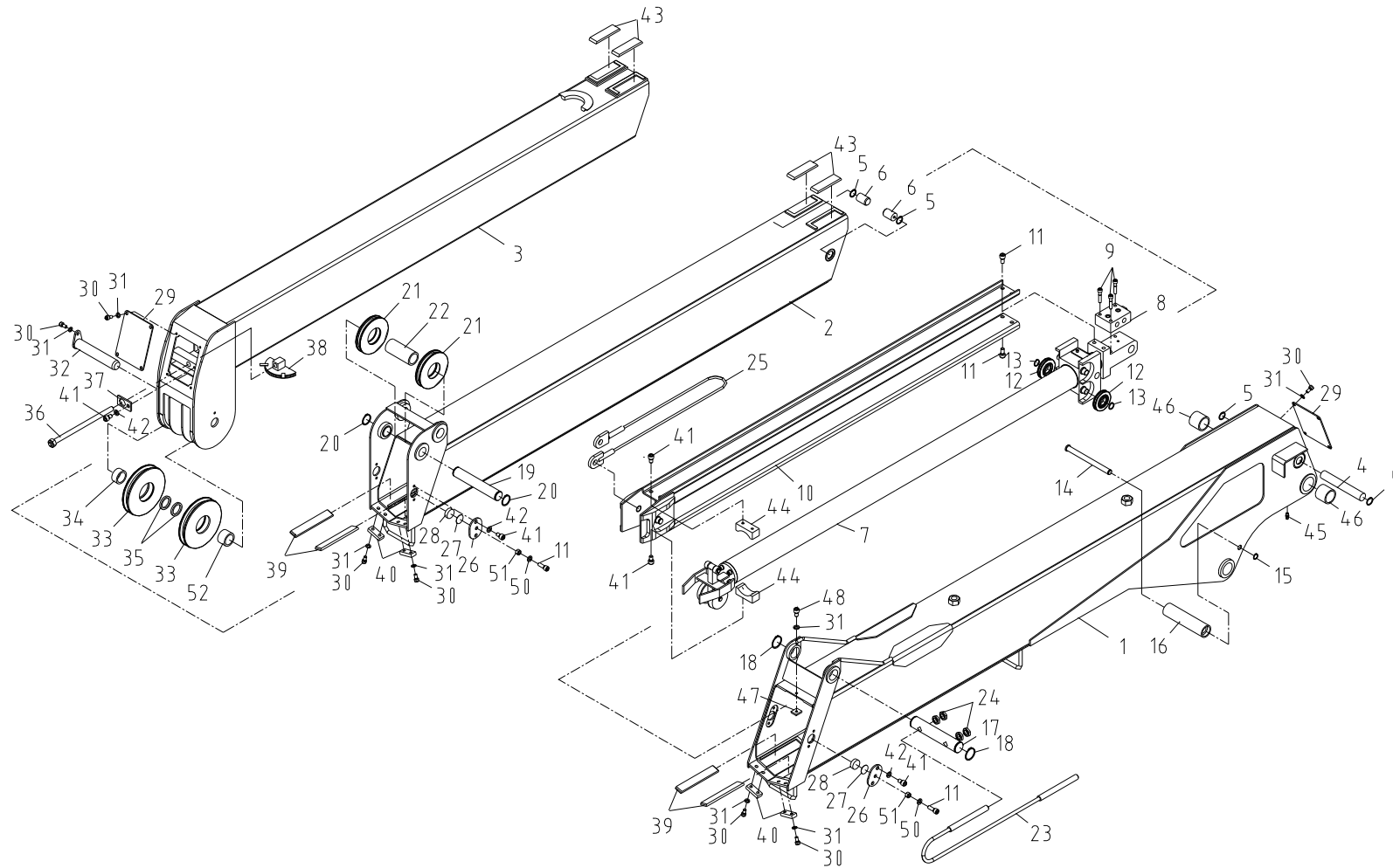
붐 조립체 Fig. 1 SCS263 BOOM ASS'Y
