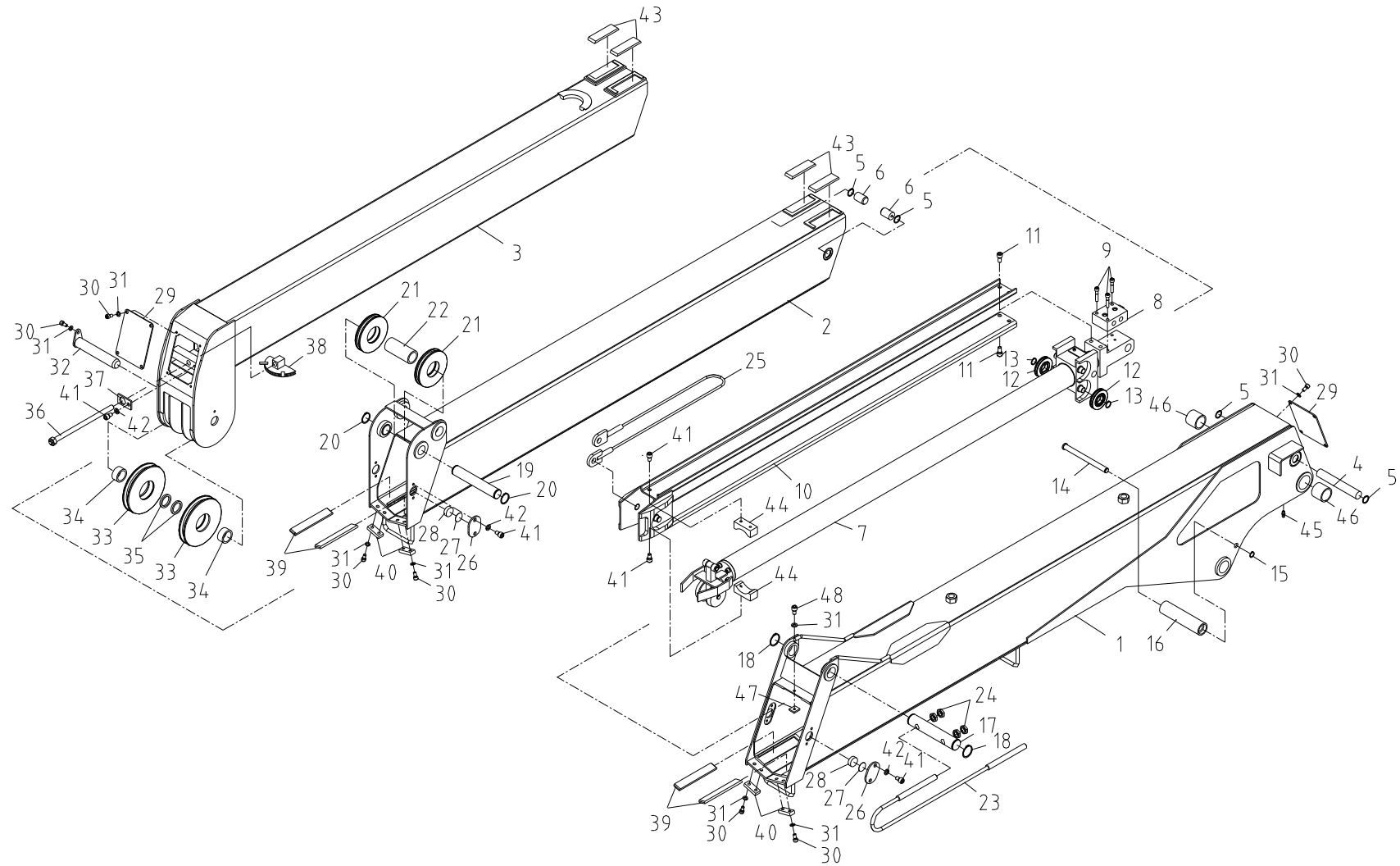
붐 조립체 Fig. 1 SCS263 BOOM ASS'Y
