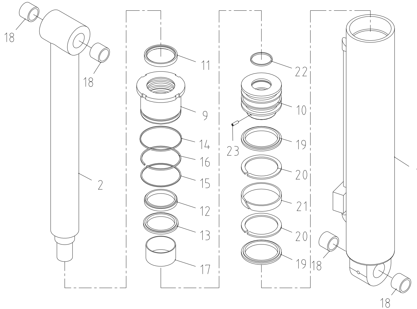
데릭 실린더 조립체 Fig. 2-1 SCS263 DERRICK CYL' ASS'Y
