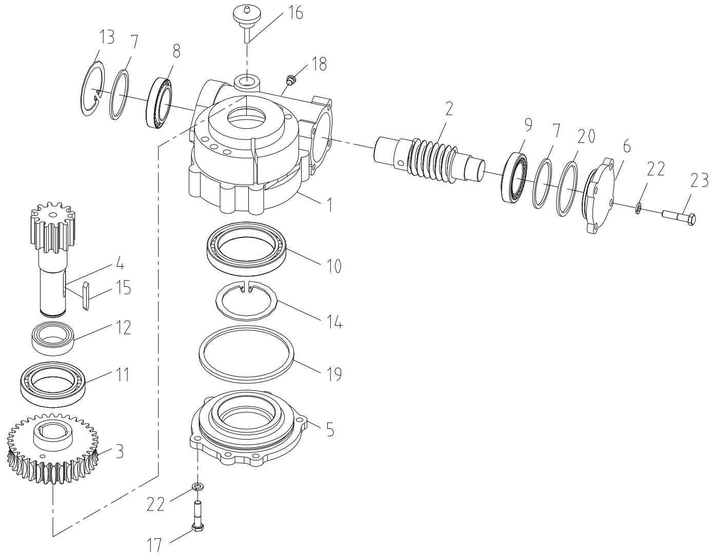
스윙 감속기 조립체 Fig. 3-2 SCS263 SWING R/G ASS'Y
