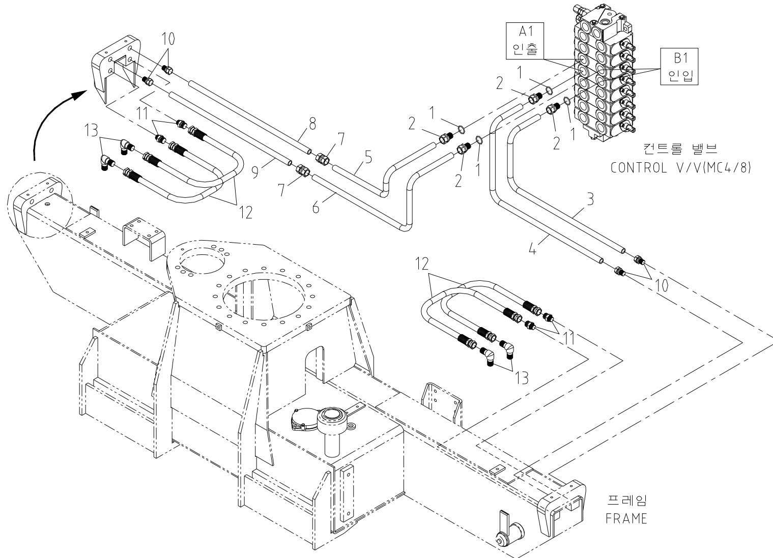
아우트리거 배관 Fig. 5-6 SCS263 OUTRIGGER PIPING
