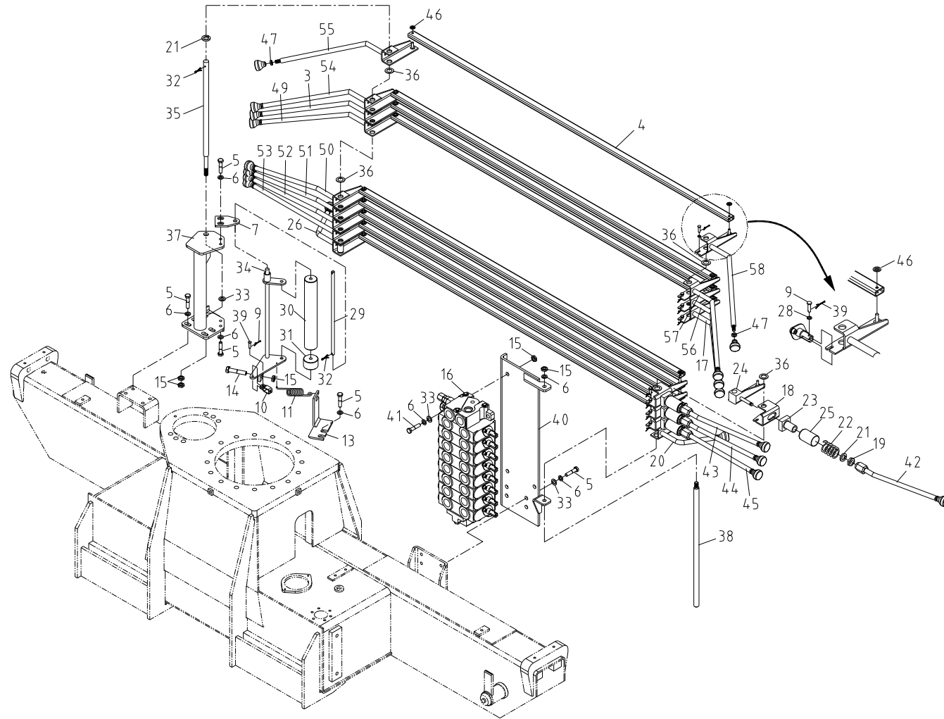
오퍼레이션 조립체 Fig. 3-4 SCS263 OPERATION ASS'Y
