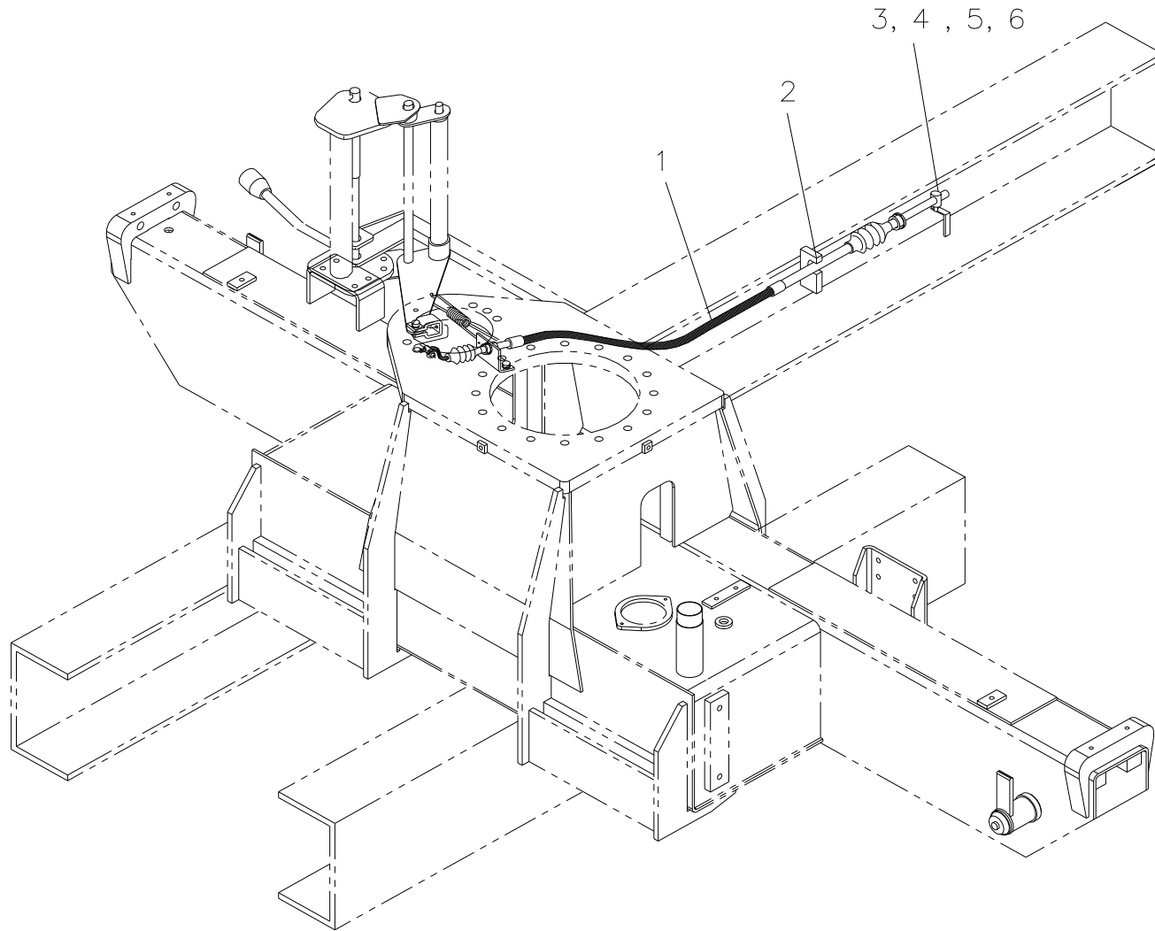
악셀 시스템 파트 Fig. 8-3 SCS263 ACC' SYSTEM PART
