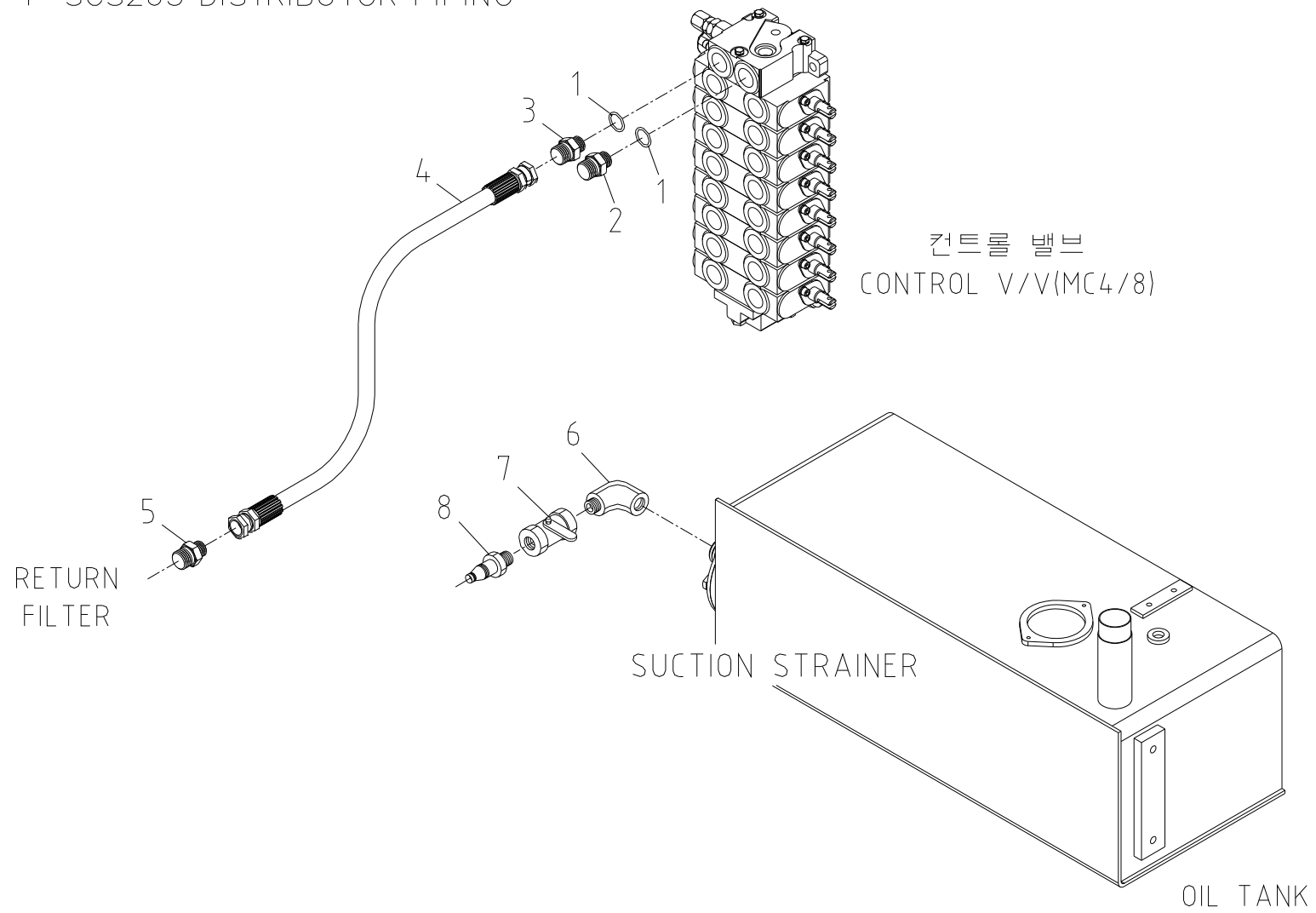
디스트리뷰터 배관 Fig. 5-1 SCS263 DISTRIBUTOR PIPING
